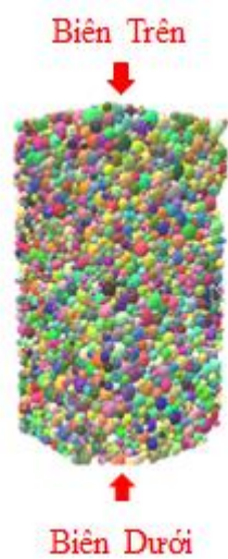
Hình 5.7: Điều kiện biên của thí nghiệm kéo, nén
