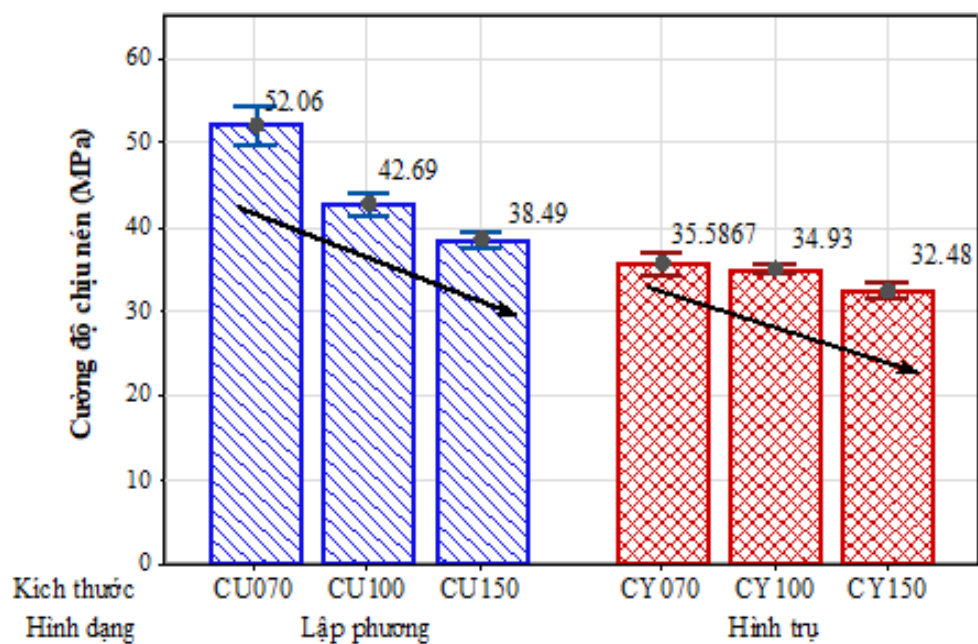
(b) Cường độ chịu nén
