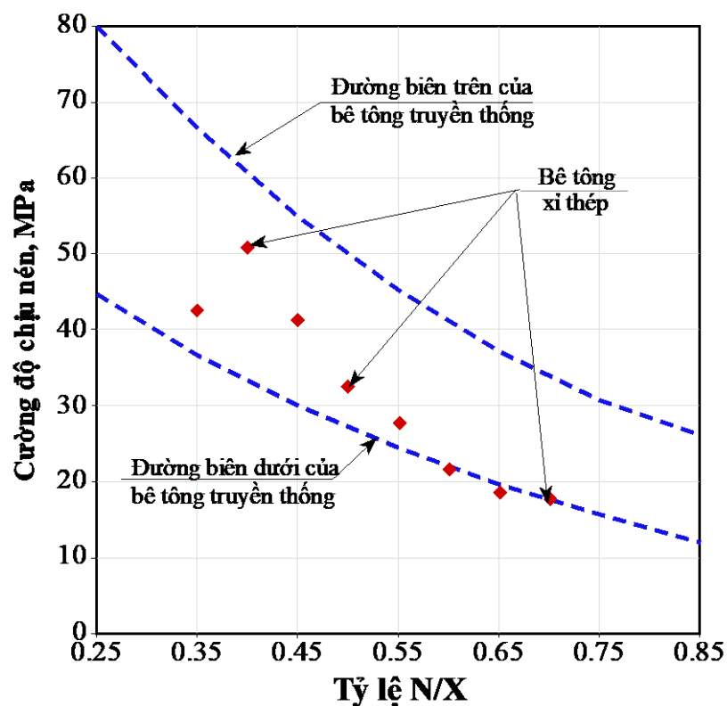
Hình 3.20: Quan hệ giữa cường độ chịu nén và tỷ lệ X/N của BTXT và bê tông truyền thống, sử dụng mẫu trụ 150 \times 300 mm [105]
