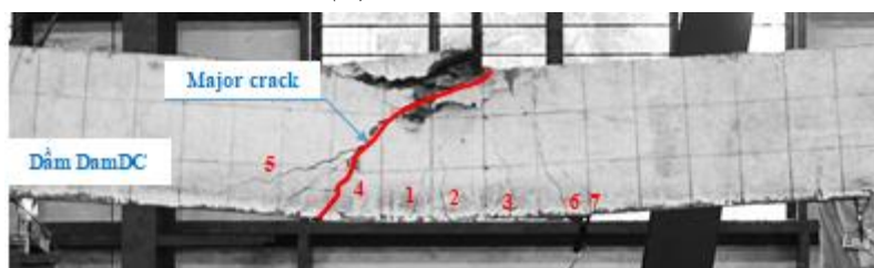
(d) Dầm DamDC [137]
